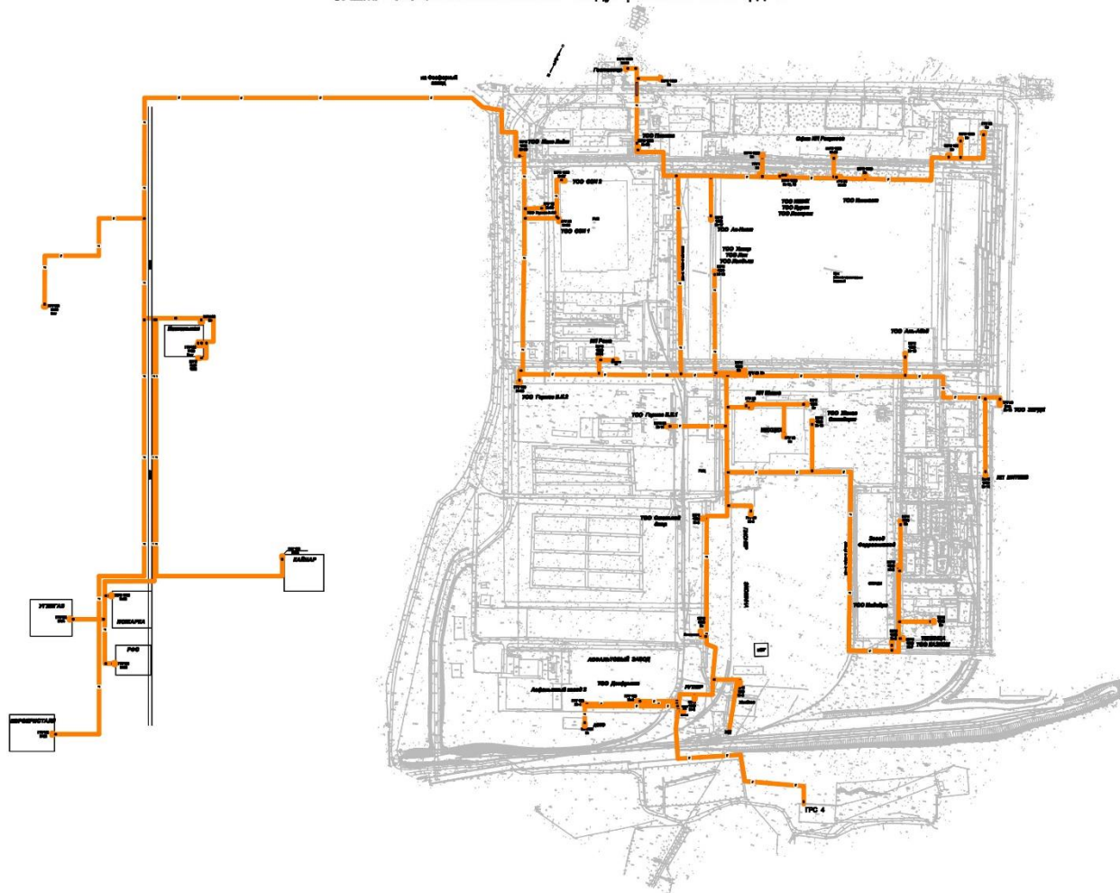
СХЕМА системы газоснабжения "Индустриальной зоны Ордабасы"
